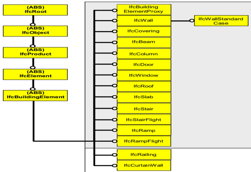
Fig. 1 IFC hierarchy
