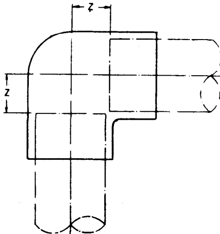
FIG. 1 99° ELBOW
