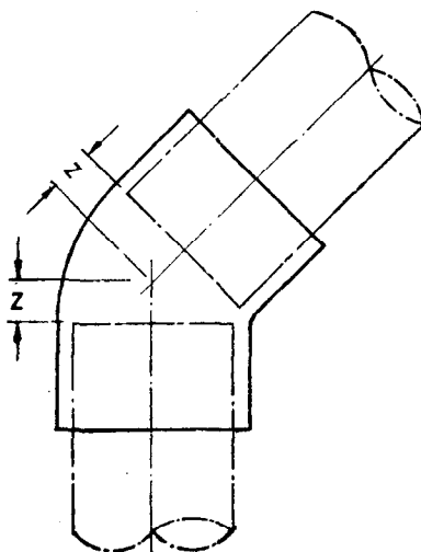
FIG. 1 45° Elbow
