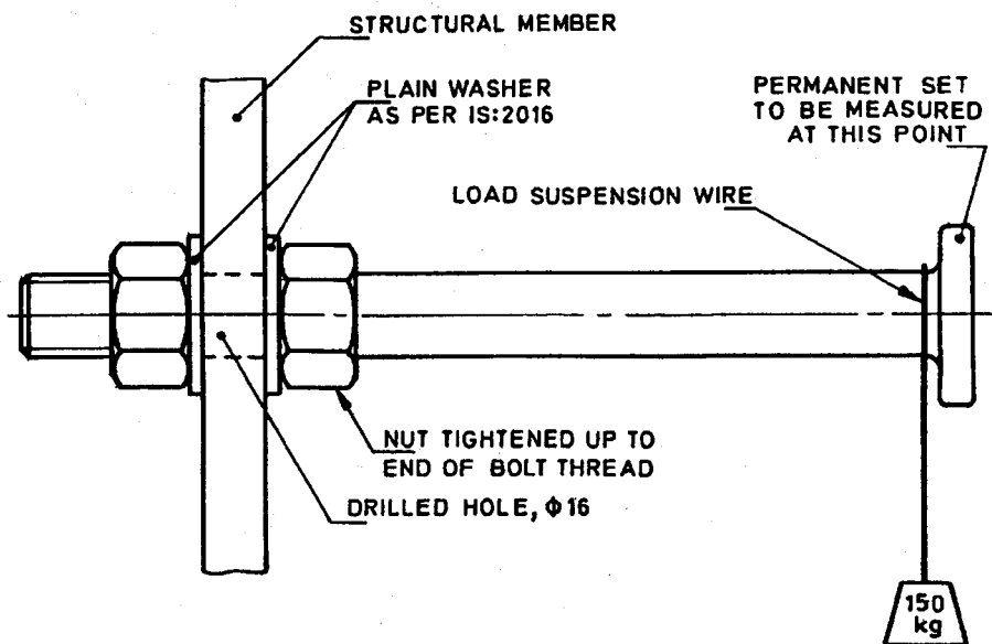
FIG. 2 CANTILEVER TEST
